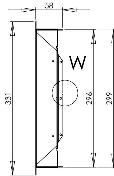
SECTION V-V
